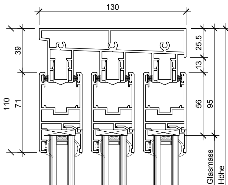
Deckenschiene 3-gleisig
